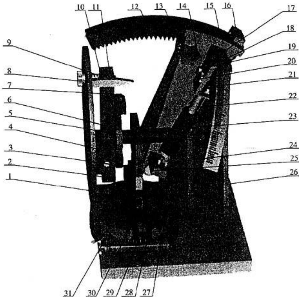
图 A.1 车轮定位角模拟机构
